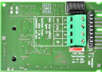
EE850-M1xJ3
