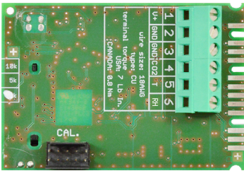
EE850-M12
